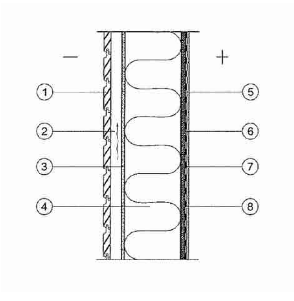
US 02b Pesemisruumi puitvälissein, laudkate. Lihtne seinakarkass
